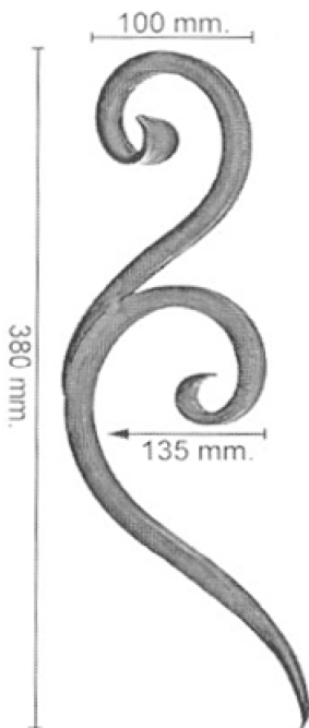
Quadro 14x14 H.380xL.135mm RIF 174
