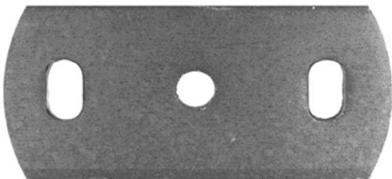
H.60 X L.120mm Sp.8mm SAV 25 foroø12 fori 20x11
