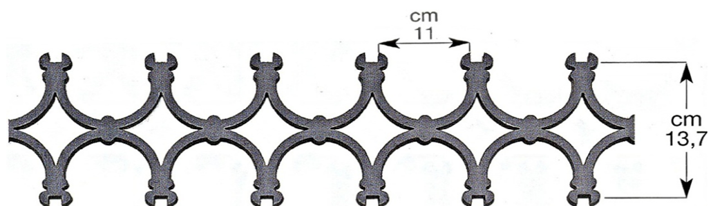
SAL 23 L. 200cm Spessore 10mm
