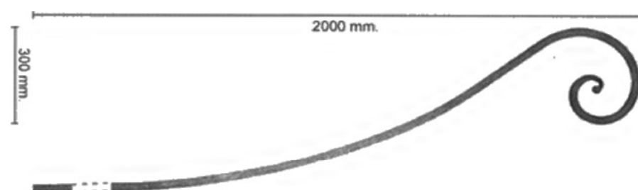
MARTELLATO SINISTRO ≠ 35x8mm CIM 40
