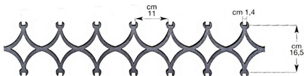
SAL 13 L. 200cm Spessore 10mm
