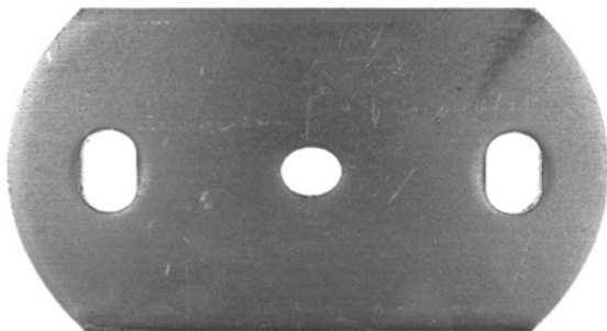
H.80 X L.120mm Sp.8mm SAV 26 foroø12 fori 20x11
